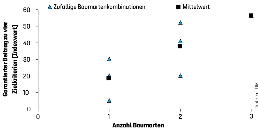
Abb. 3: Garantierter Beitrag zu vier Zielkriterien bei unterschiedlicher Anzahl an verfügbaren Baumarten auf der Bestandesebene. Zur Auswahl standen Tanne, Fichte und Buche.
